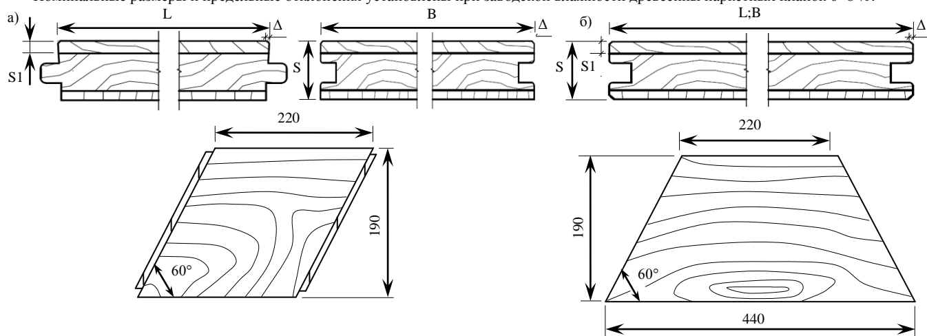
Рисунок 1: а) продольный и поперечный профили и внешний вид паркета типа ТЕ03 «Ромб» с углом \alpha = 60^\circ ; б) продольный и поперечный профили и внешний вид паркета типа ТЕ03 «Трапеция» с углом \alpha = 60^\circ
