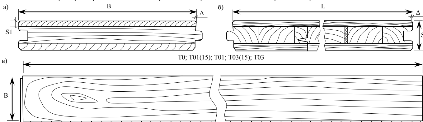
Рисунок 1: а) поперечный профиль конструкции «Т» с замком типа T&G (паз – гребень); б) продольный профиль конструкции «Т» с замком типа T&G (паз – гребень); в) внешний вид паркета типа T0; T01(15); T01; T03(15); T03.
