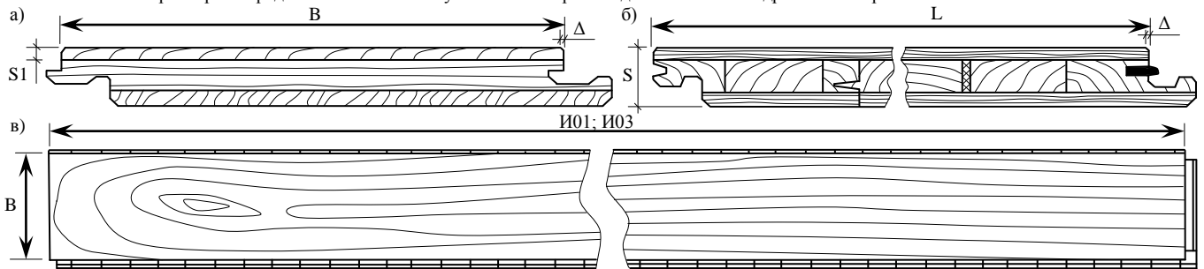
Рисунок 1: а) поперечный профиль конструкции «И» с замком типа CosLoc; б) продольный профиль конструкции «И» с замком типа CosLoc; в) внешний вид паркета типа И01, И03
